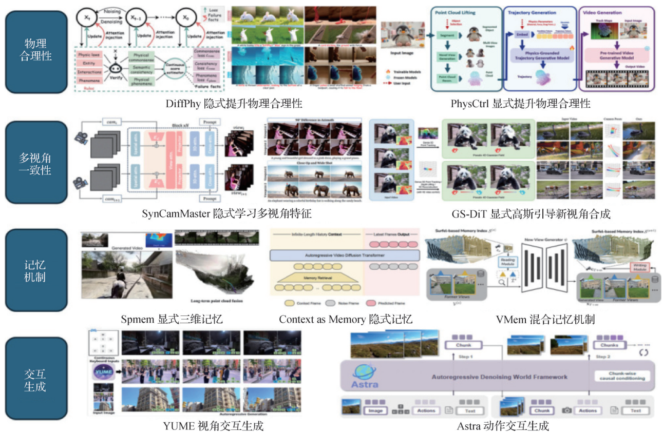
图7 视频世界模型2025年代表性工作 Fig. 7 Representative works on video world models in 2025
